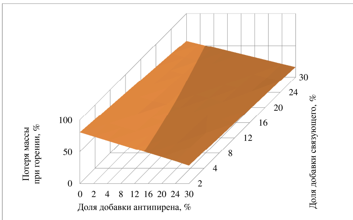
Рисунок 6.11 – Зависимость потери массы при горении от доли добавки алюмохрофосфатного связующего и антипирена Al(OH)_3 для композита без мягких отходов древесины
