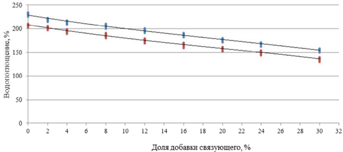
Рисунок 4.3 – Зависимость водопоглощения от массовых долей добавки фенолформальдегидного связующего, где \bullet – для плит из хлопка, \bullet – для плит из льна
