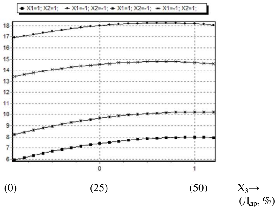
Рисунок 4.13 – График зависимости разбухания по толщине за 24 часа от доли добавки отходов древесины
