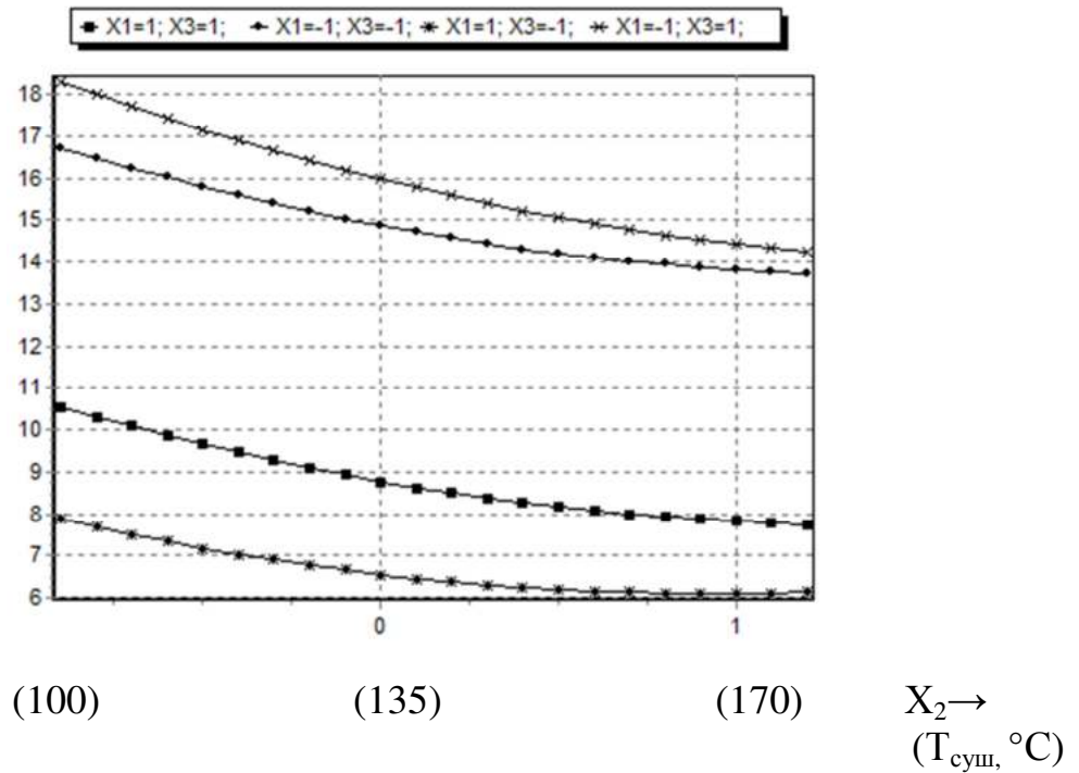
Рисунок 4.12 – График зависимости разбухания по толщине за 24 часа от температуры сушки
