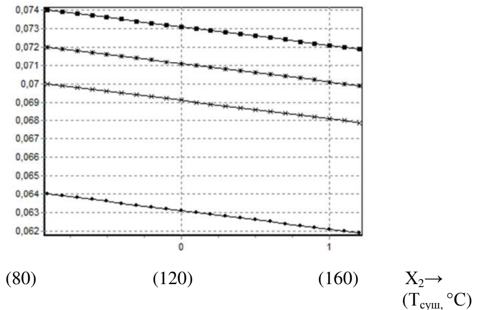
Рисунок 6.13 – График зависимости коэффициента теплопроводности от температуры сушки
