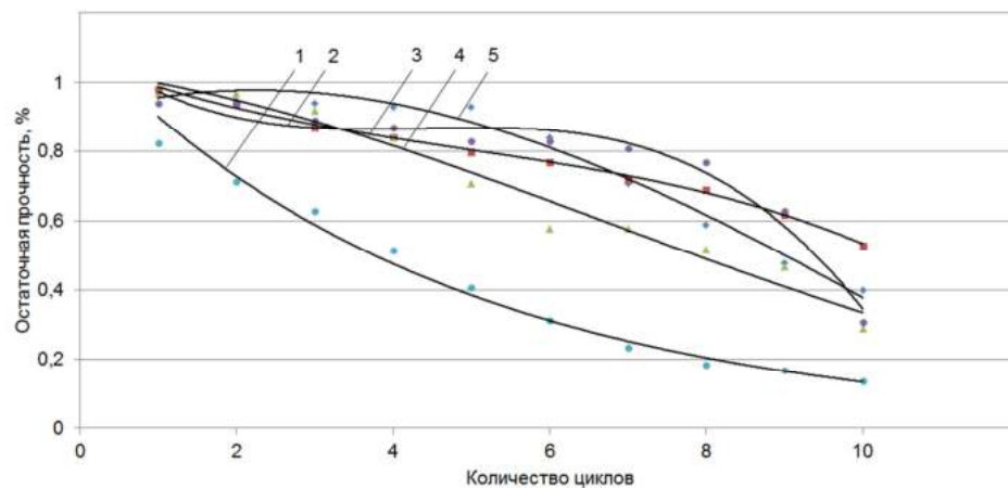
Рисунок 4.5 – Зависимости остаточной прочности при статическом изгибе, % для плит из отходов хлопка после циклов температурно-влажностных воздействий: 1 – ДСтП на ФФС; 2 – композит из хлопка на АХФ; 3 – композит из хлопка на ЖС; 4 – композит из хлопка на КФС; 5 – композит из хлопка на ФФС
