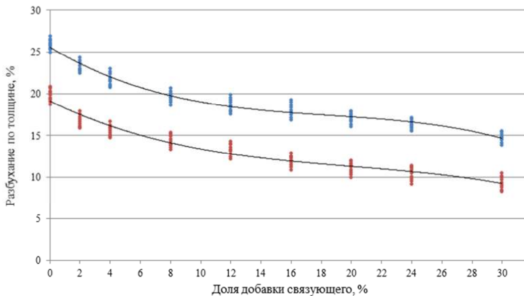
Рисунок 4.2 – Зависимость разбухания по толщине от массовых долей добавки фенолформальдегидного связующего, где * – для плит из хлопка, * – для плит из льна
