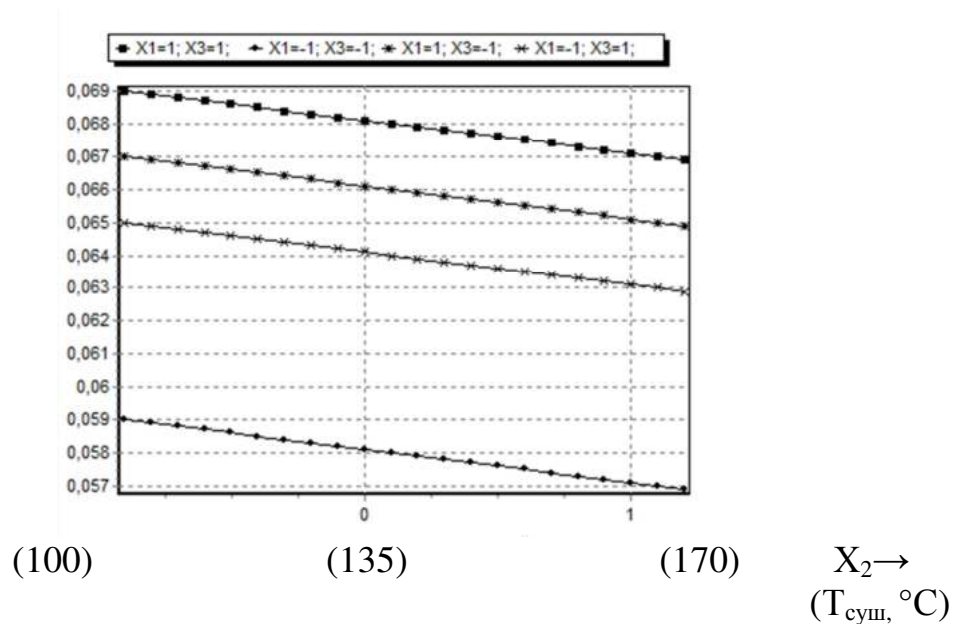
Рисунок 5.8 – График зависимости коэффициента теплопроводности от температуры сушки
