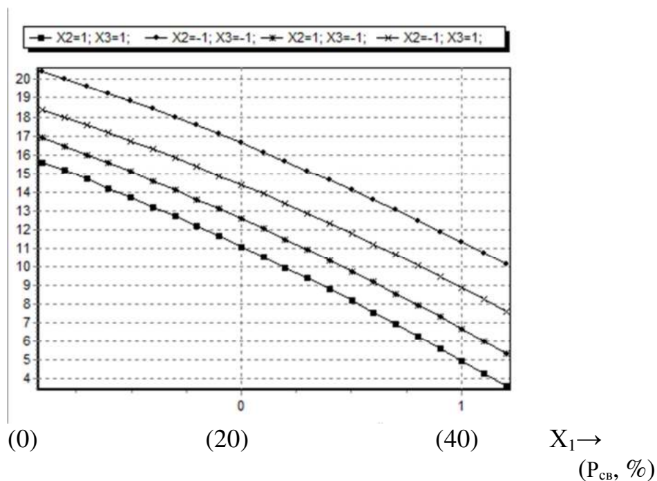
Рисунок 6.18 – График зависимости разбухания по толщине за 24 часа от доли добавки связующего
