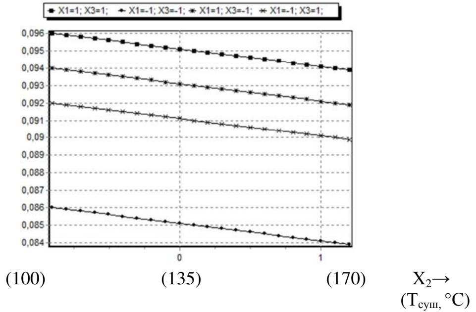
Рисунок 5.26 – График зависимости коэффициента теплопроводности от температуры сушки
